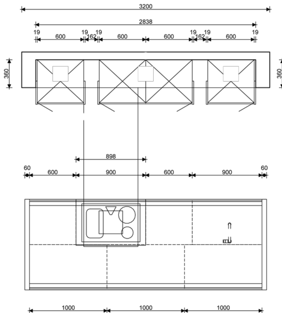
Cuisine d'exposition FR- MK-01
